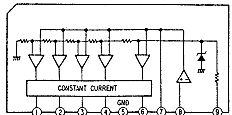
IC951, 971 IR2E31A
